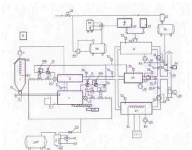
Tehnološka shema za spaljivanje životinjskog otpada - Trigeneracija (CHCP)
