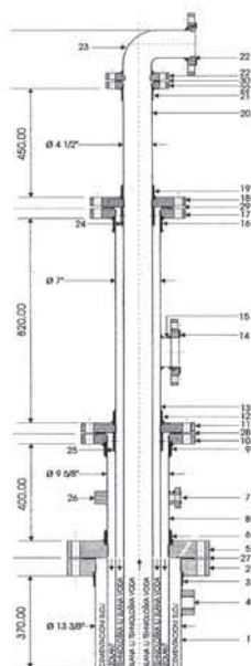
slika 1. Sklopni crtež
