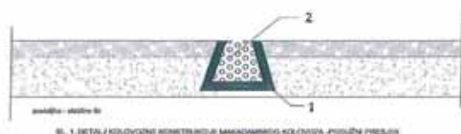
SL. 1. BETALNI KOLVOZNE KONSTRUKCIJE I MAKADAMSKI KOLVOZ - PODUŽNI PRESJEK
