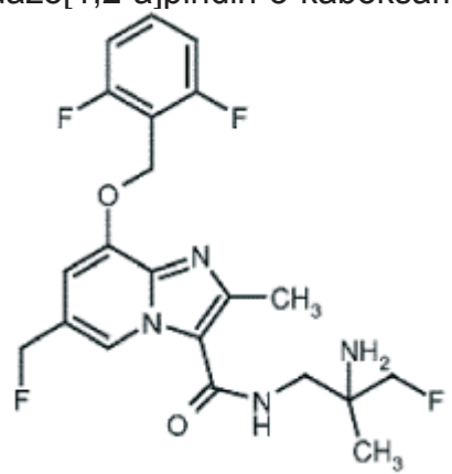
ent -N-(2-amino-3-fluoro-2-metilpropil)-8-[(2,6-difluorobenzil)oksi]-6-(fluorometil)-2-metilimidazo[1,2-a]piridin-3-kaboksamid
