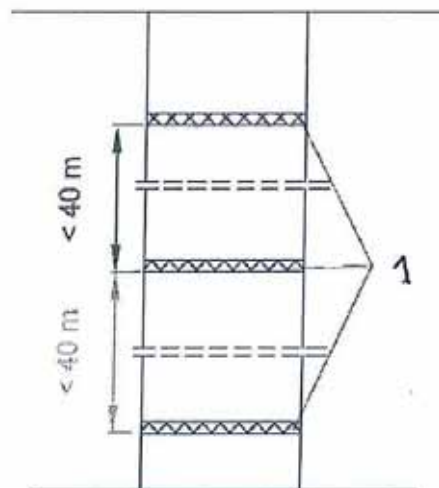
SL. 2. MAKADAMSKI PUT SA USPONOM I PROPUSNIM TRAKAMA
