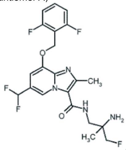
ent -N-(2-amino-3-fluoro-2-metilpropil)-8-[(2,6-difluorobenzil)oksi]-6-(fluorometil)-2-metilimidazo[1,2-a]piridin-3-kaboksamid
