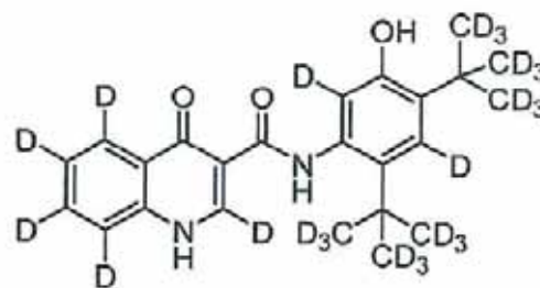
Jedinjenje 100
