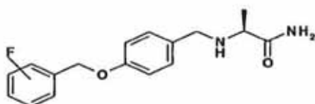
safinamide (Ia): 3-F
